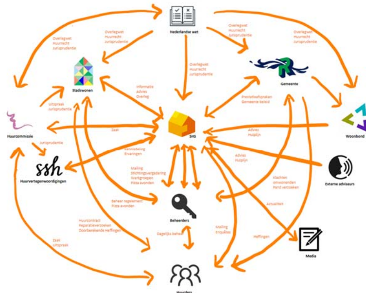
Figuur 3. Netwerflow
